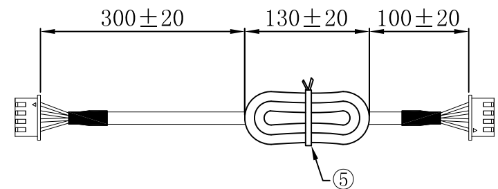
扎线示图
